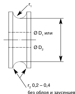
Рис. 2.21 Радиус посадочной канавки
