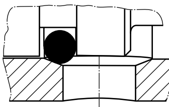
Рис. 2.27 Наилучшим решением является балансировочный паз в зоне отверстия. Уплотнительное кольцо может быть разжато и направлено через паз по входным и выходным фаскам.
