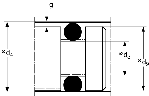
Рис. 8.35 Максимальный радиальный ход
