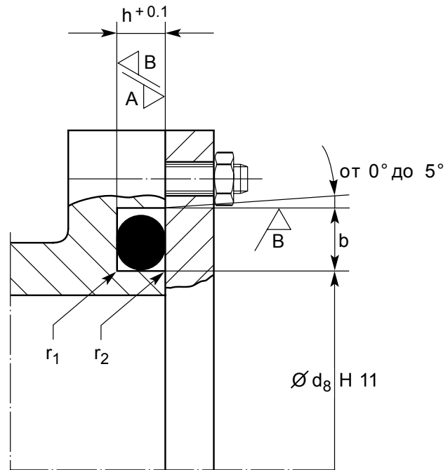
Рис. 2.9 Давление снаружи
