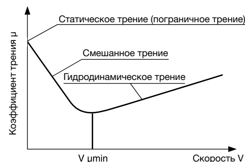
Рис. 8.18 Кривая Штрибека
