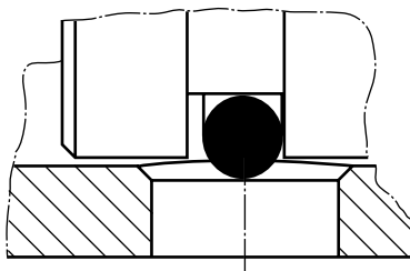
Рис. 2.26 Если изменение положения невозможно, рекомендуется использование внутренней фаски.
