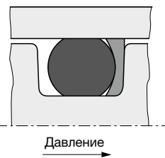
Рис. 10.4 Антиэкструзионное кольцо на стороне без давления предотвращает выдавливание в зазор.
