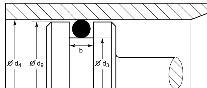
Рис. 3.9 Уплотнение поршня и радиальное сжатие
