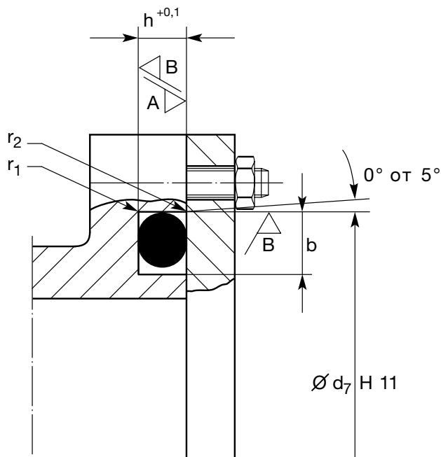
Рис. 2.8 Давление изнутри
