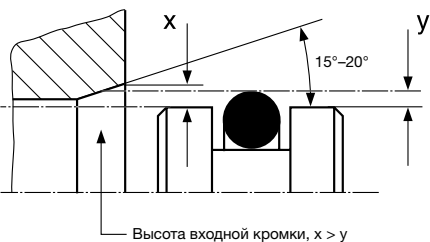
Рис. 2.24 На схеме показана фаска входной кромки и уплотнительное кольцо перед сжатием. Размер «x» должен быть больше размера «y» для обеспечения сборки без помех.
