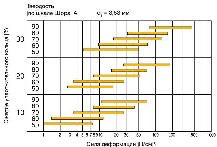
1) Длина окружности уплотнительного кольца (см). Рис. 8.28
