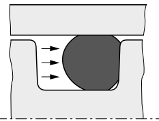
Рис. 10.2 При подаче давления уплотнительное кольцо действует как несжимаемая жидкость, прилагая давление на канавку пропорционально давлению системы.
