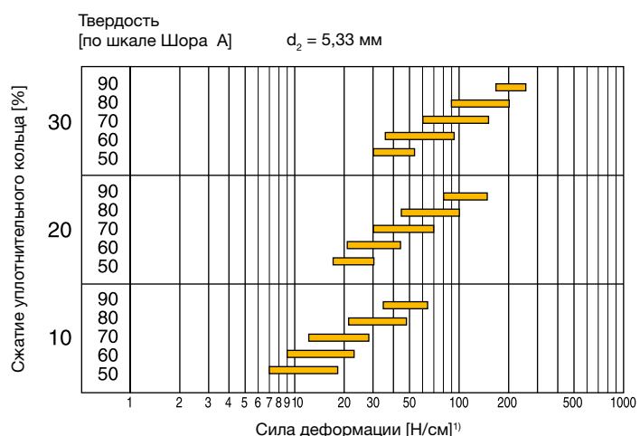
1) Длина окружности уплотнительного кольца (см). Рис. 8.29
