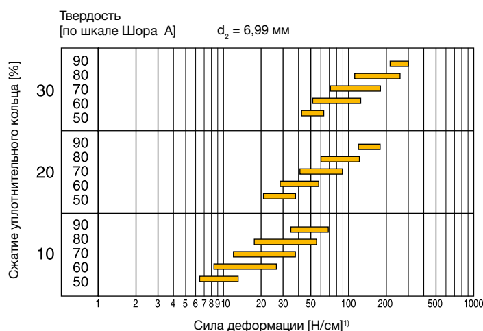
1) Длина окружности уплотнительного кольца (см). Рис. 8.30
