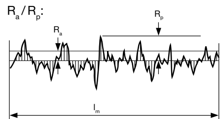
Рис. 8.15 Терминология шероховатости
