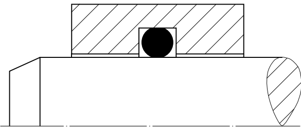
Рис. 2.1 Внутренняя посадочная канавка («уплотнение штока»): уплотнительное кольцо с радиальным сжатием
