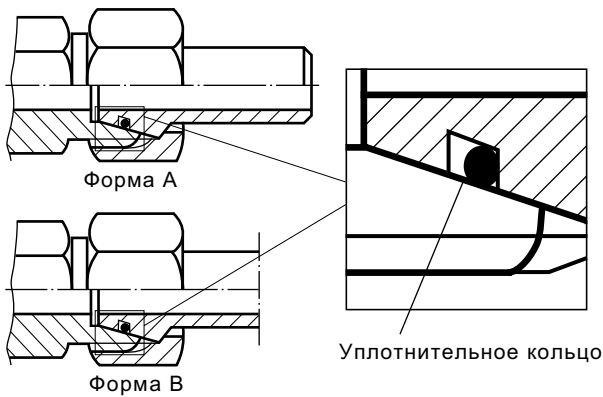
Рис. 4.4 Сборка
