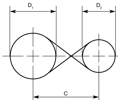
Рис. 2.20 Перекрестное исполнение
