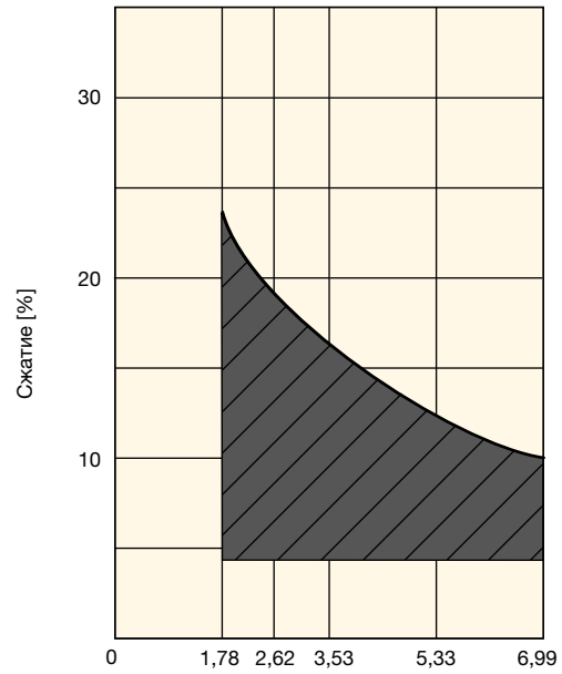
Поперечное сечение уплотнительного кольца d_2 [мм]
